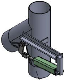
VALVULA 3 VIAS 2 POSIÇÕES COM ACIONAMENTO PNEUMÁTICO
