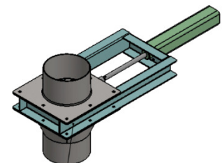
VALVULA DE GUILHOTINA COM ACIONAMENTO PNEUMÁTICO
