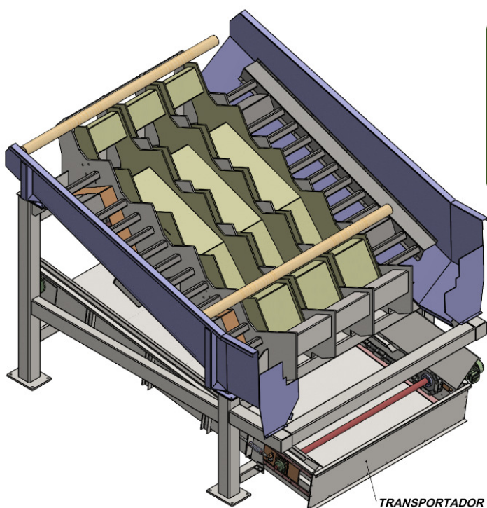
TRANSPORTADOR TIPO REDLER PARA OS RESÍDUOS
