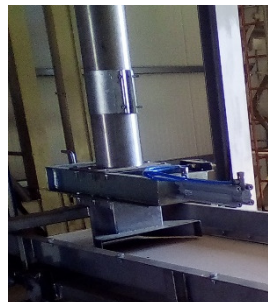
VALVULA DE GUILHOTINA MOTORIZADA DE ALTURA REDUZIDA
