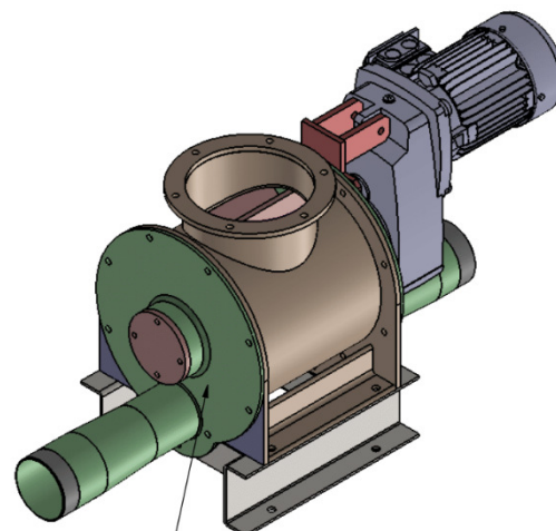
ECLUSA \varnothing 300 PARA TRANSPORTE PNEUMÁTICO
