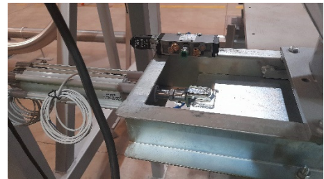
VALVULA DE GUILHOTINA MOTORIZADA DE PRECISÃO COM ENCODER
